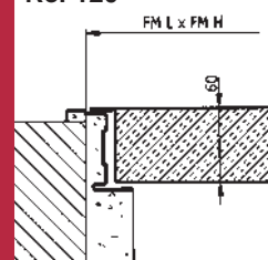
Particolare Porta UNIVER REI 120
